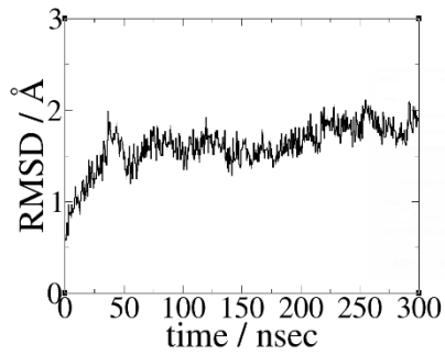
(b) docking pose2
