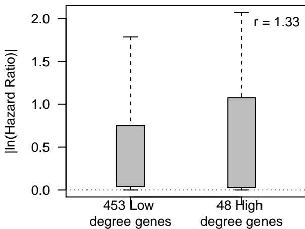
UCEC DSS
