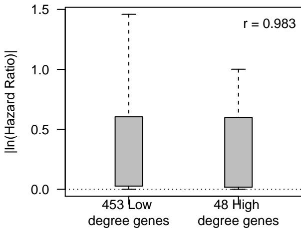
UCEC OS
