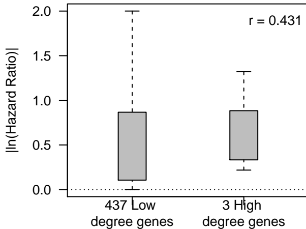
KIRC PFI
