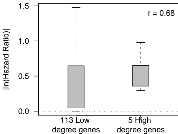
LGG DSS
