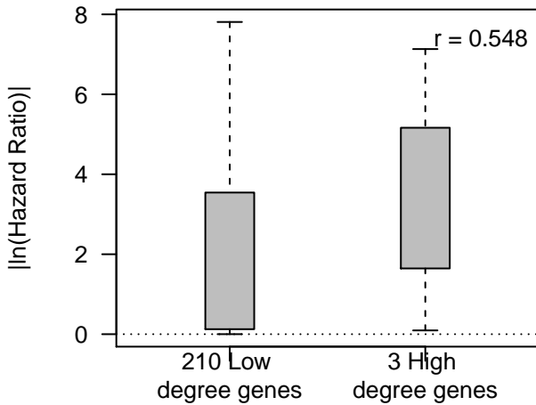
DLBC OS
