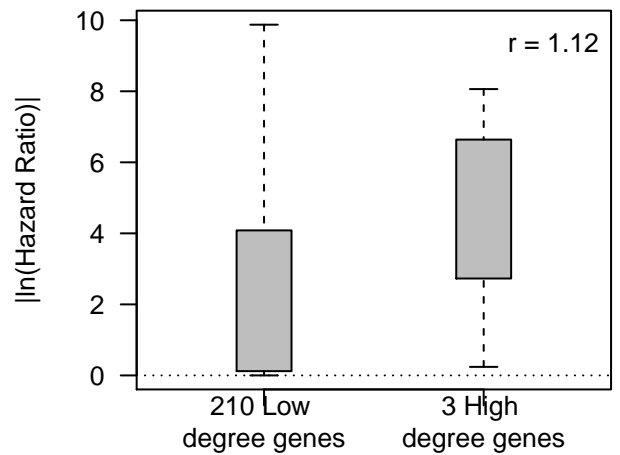
DLBC PFI
