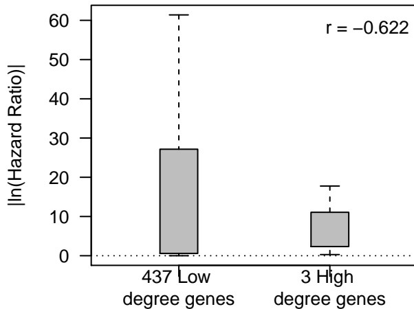
KIRC DFI
