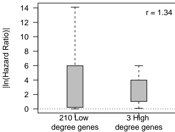
DLBC DSS
