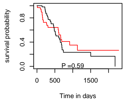
OS hsa-mir-3687
