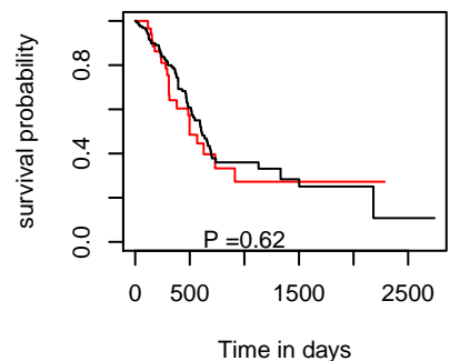
OS hsa-mir-4763
