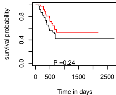
DSS hsa-mir-9-2
