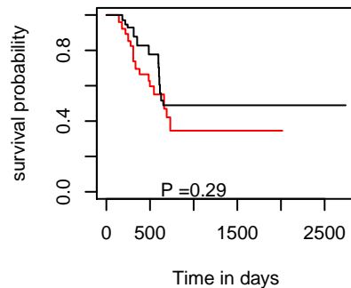
DSS hsa-mir-93
