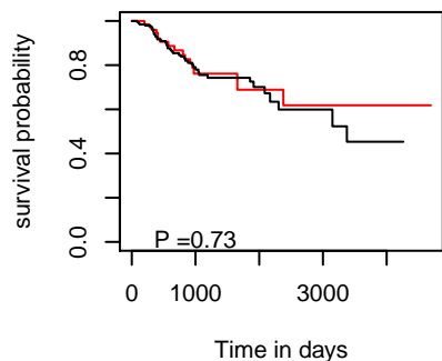
DSS hsa-mir-3618
