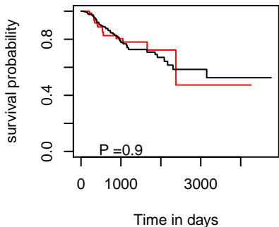
DSS hsa-mir-4763
