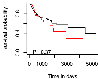
PFI hsa-mir-548d-1
