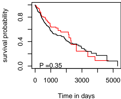
OS hsa-mir-3926-2
