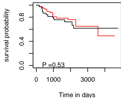
DSS hsa-mir-185
