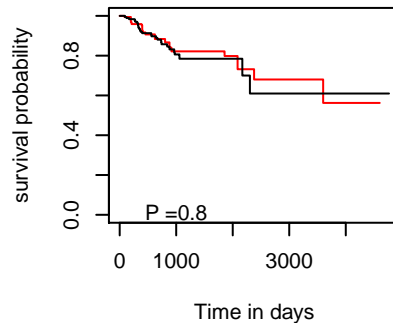
DSS hsa-mir-4707
