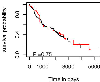
OS hsa-mir-4492
