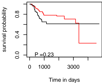
DSS hsa-mir-130b
