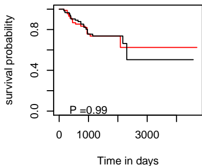
DSS hsa-mir-3678
