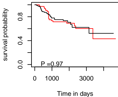
DSS hsa-mir-4492
