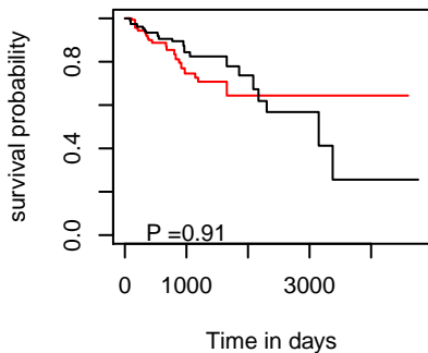
DSS hsa-mir-7-2
