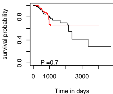
DSS hsa-mir-30d
