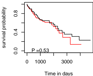
OS hsa-mir-887
