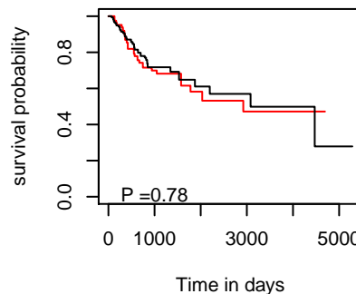
PFI hsa-mir-4444-2
