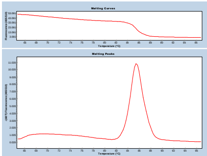
NAPE-PLD
