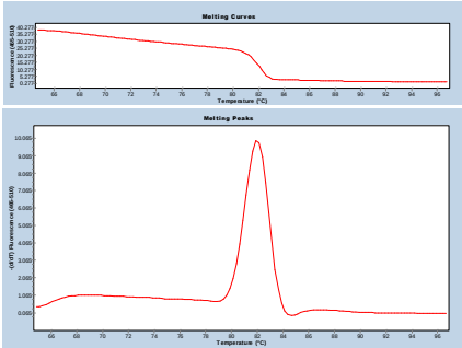
IL-6
