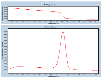
TNFα
