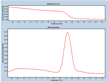
MGL
