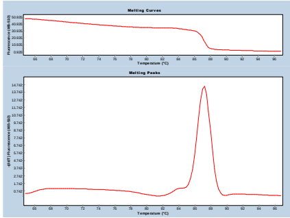
FAAH
