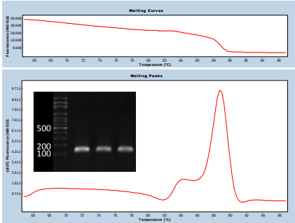
CB1R
