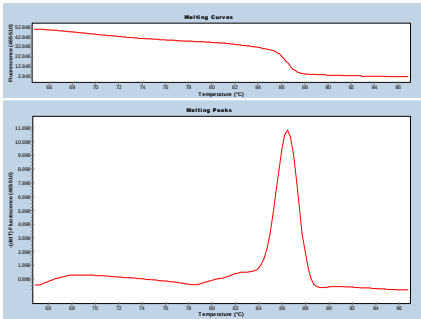
IGF-I P1
