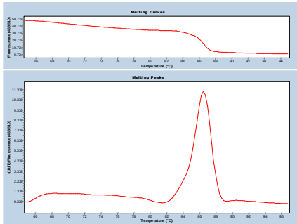
IGF-I P2
