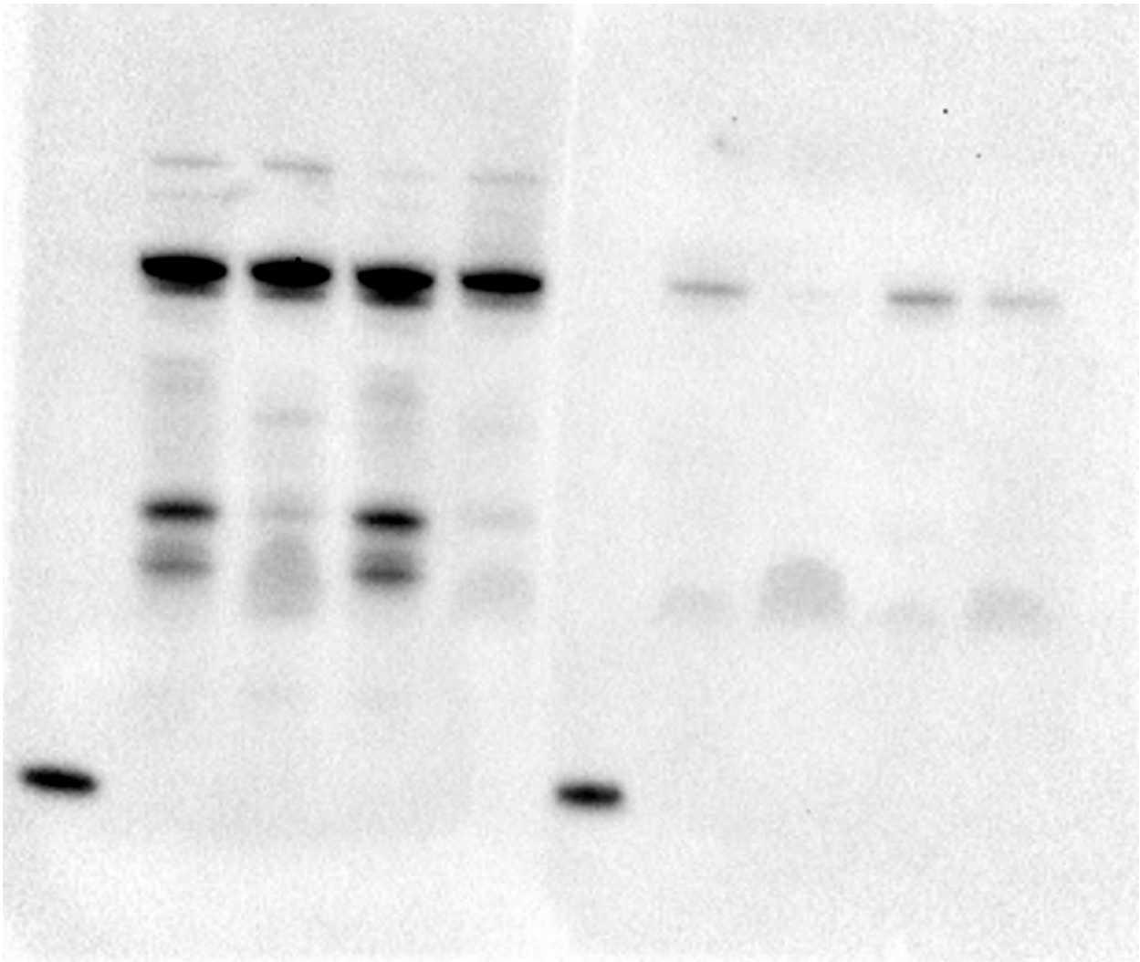
Stat3 / pStat3
